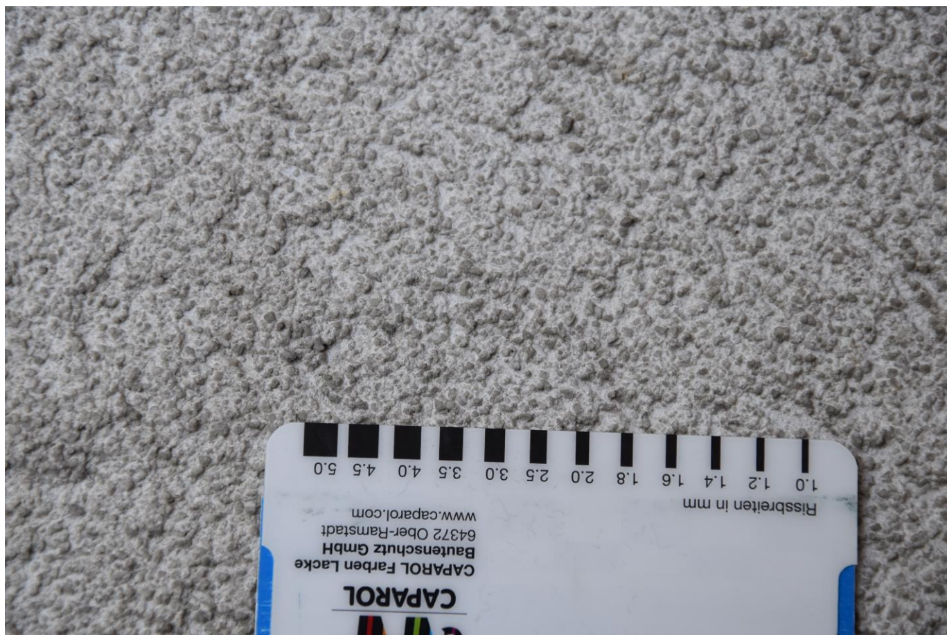
Detail - změření zrnitosti omítky 1,5 mm.
