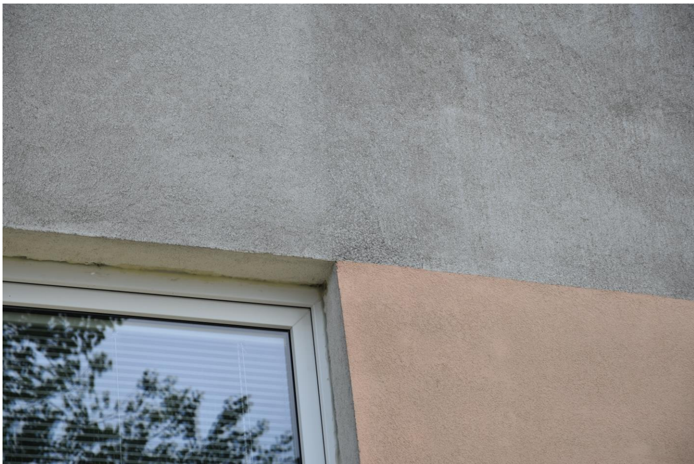
Detail – praskliny u nároží oken a nepoužití okenní připojovací lišty ( APU )
